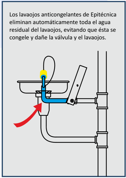
Ducha con Lavaojos Anticongelante Recomendado hasta -10°C
