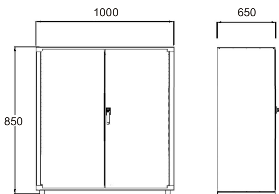
ARTICULO 7610PLA DIMENSIONES EN mm
