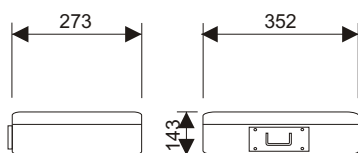
ARTICULO 7310 DIMENSIONES EN mm
