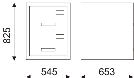
ARTICULO 7302EVO DIMENSIONES EN mm
