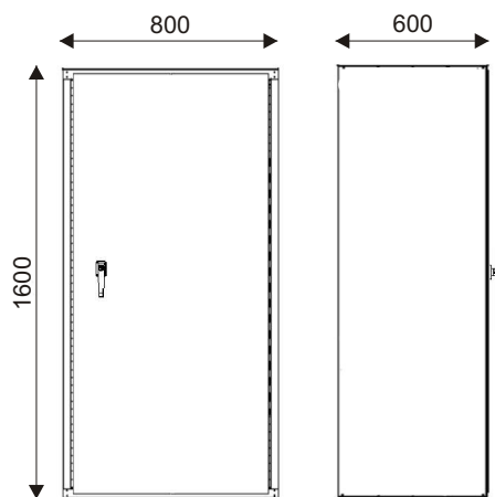
ARTICULO 7045EVO DIMENSIONES EN mm
