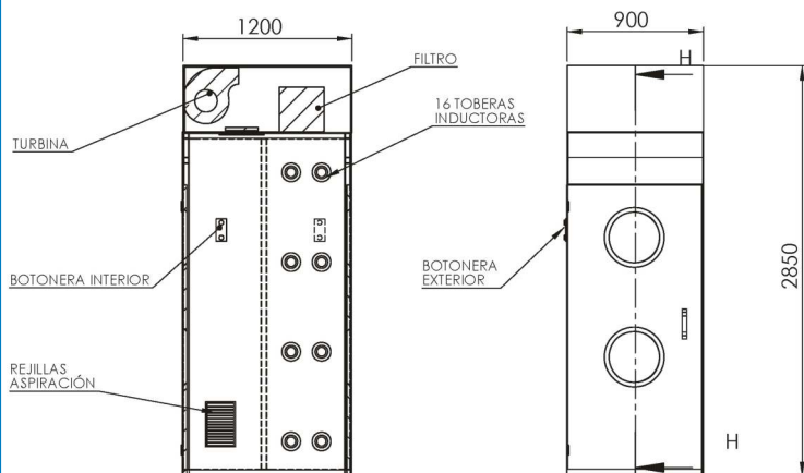
ARTICULO 6410AI DUCHA DE AIRE DIMENSIONES EN mm
