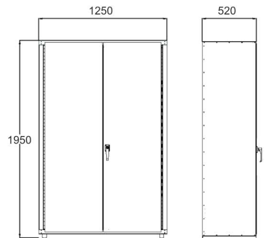
ARTICULO 7050BATM DIMENSIONES EN mm
