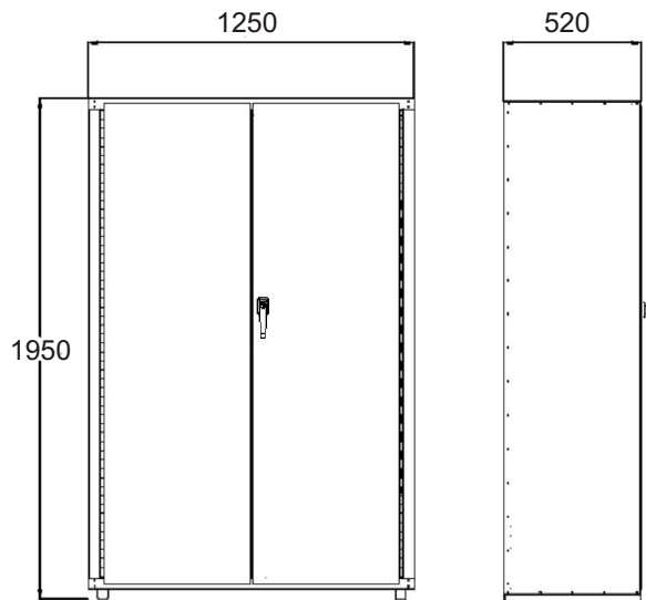
ARTICULO 7050BATM DIMENSIONES EN mm
