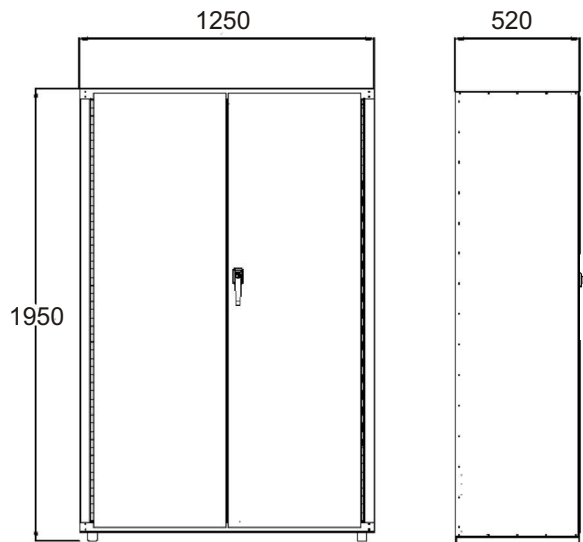
ARTICULO 7050BATA DIMENSIONES EN mm
