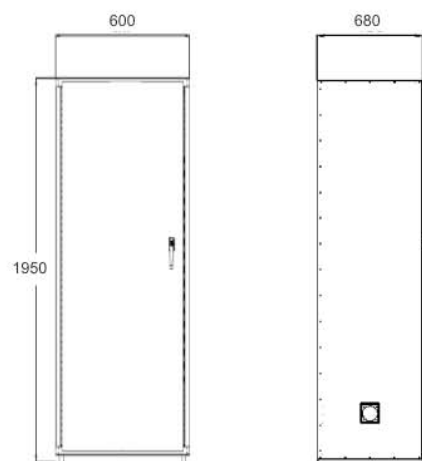
ARTICULO 7020/BAT/M DIMENSIONES EN mm
