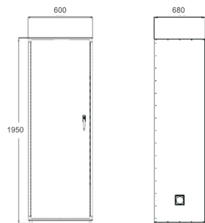
ARTICULO 7020/BAT/A DIMENSIONES EN mm
