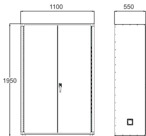
ARTICULO 7010/BAT/M DIMENSIONES EN mm
