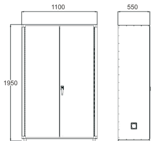
ARTICULO 7010/BAT/A DIMENSIONES EN mm
