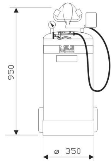
Ref. 6050-R2D2 LAVAOJOS CON DUCHA PORTATIL (50 Lts) Dimensiones en mm
