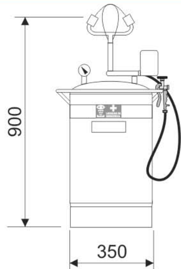
Ref. 6035-R2D2 LAVAOJOS CON DUCHA PORTATIL (32 Lts) Dimensiones en mm
