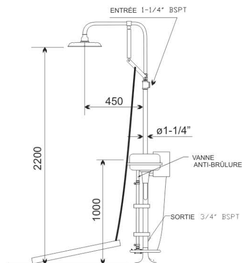
ARTICLE 6012FAE DOUCHE ET LAVE-YEUX DIMENSIONS EN mm
