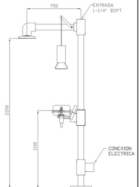
ARTICULO 6011FPHT DUCHA CON LAVAOJOS DIMENSIONES EN mm
